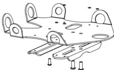
Plastique U2-204
